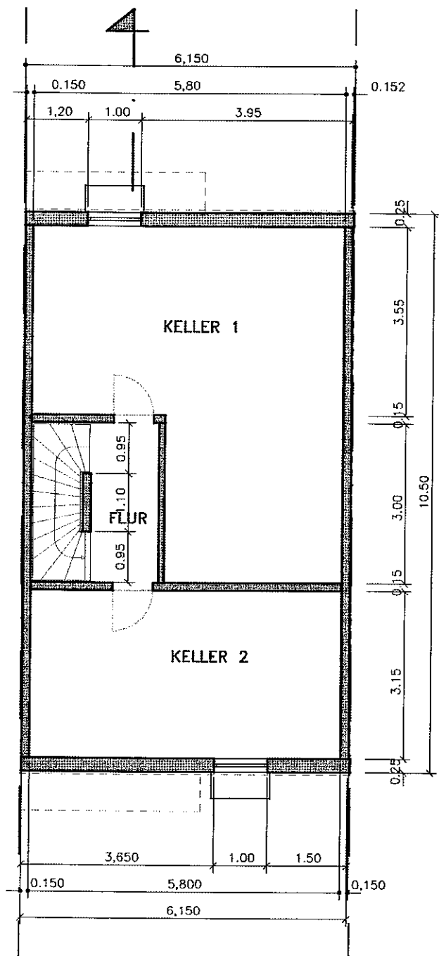
KELLERGESCHOSS
