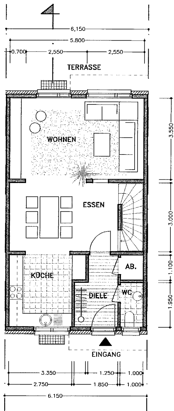
ERDGESCHOSS
