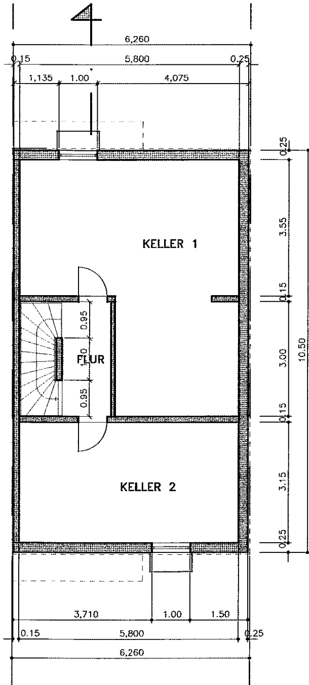
KELLERGESCHOSS
