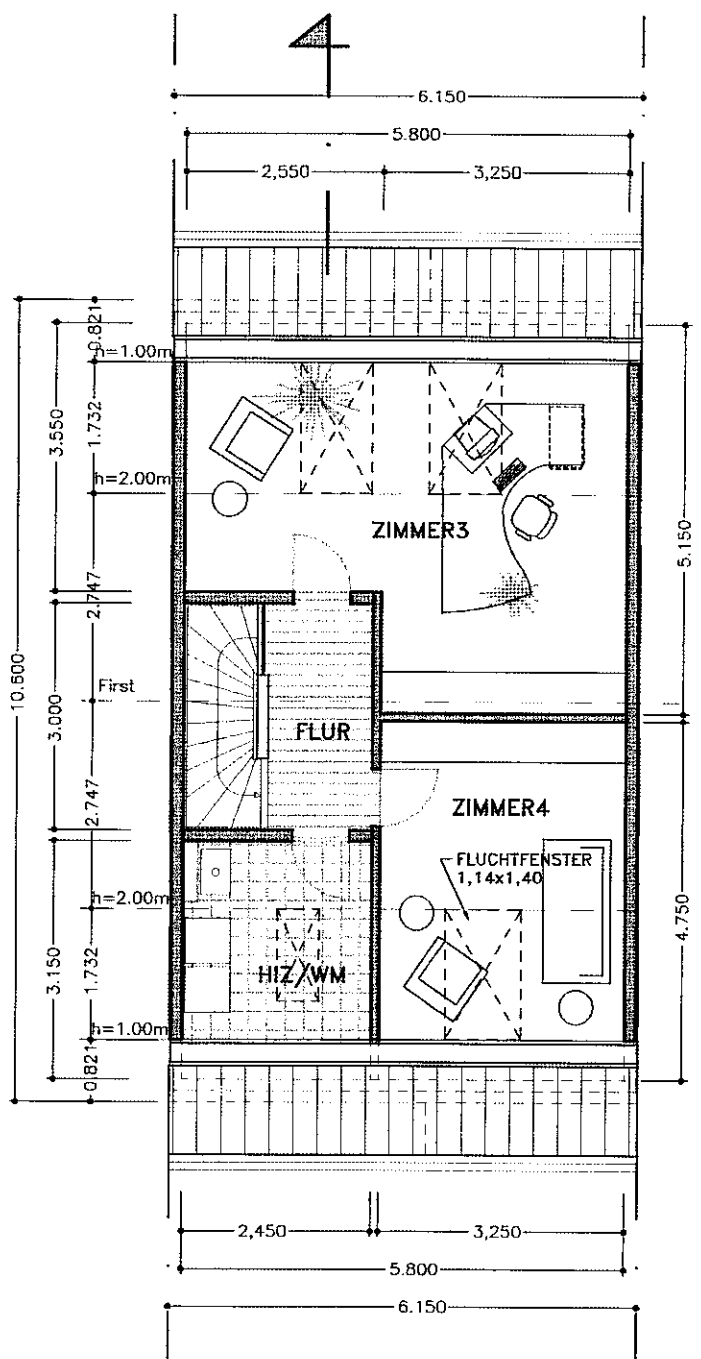
DACHGESCHOSS Sonderwunsch
