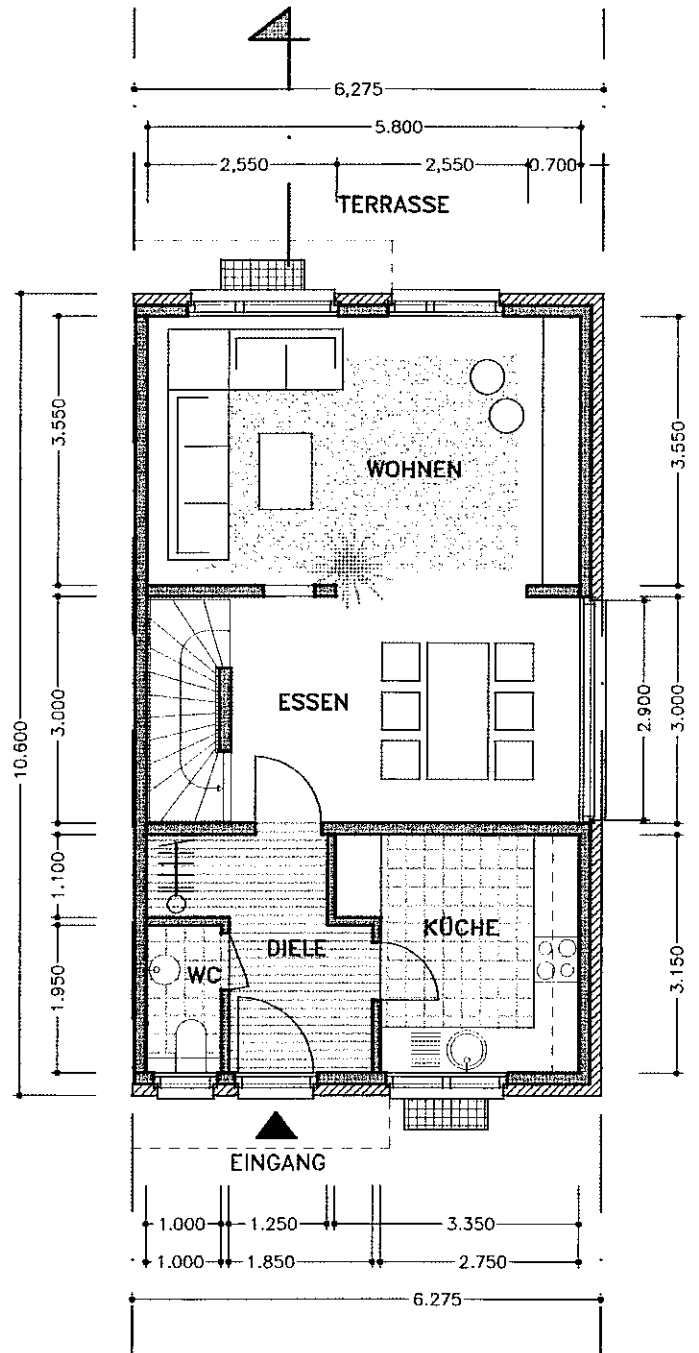
ERDGESCHOSS alternativ
