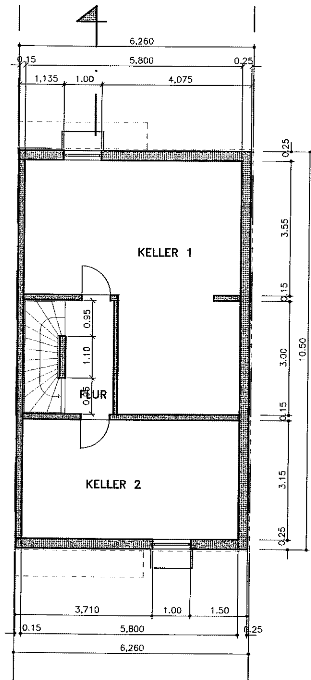
KELLERGESCHOSS
