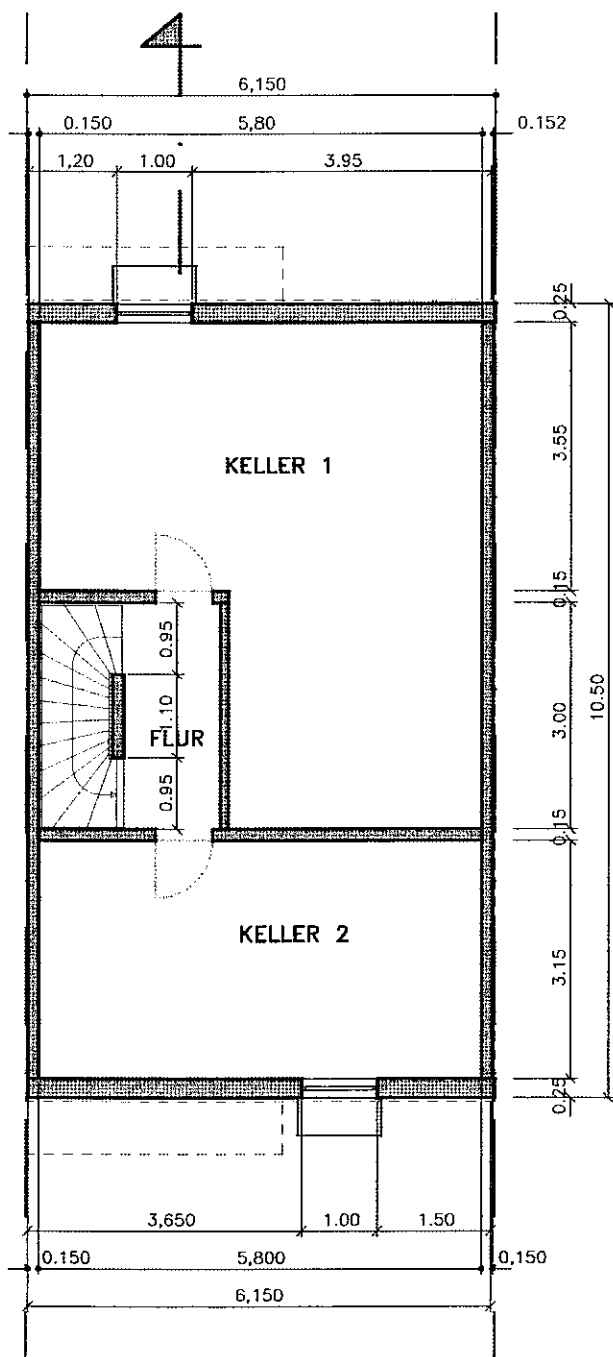
KELLERGESCHOSS
