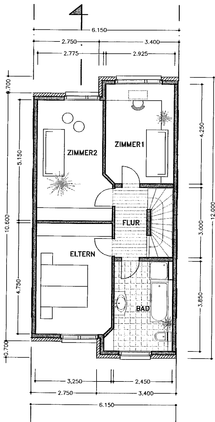
OBERGESCHOSS
