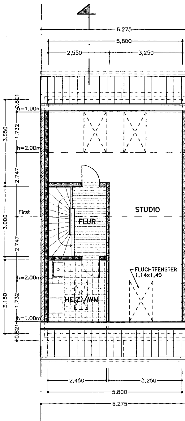
DACHGESCHOSS
