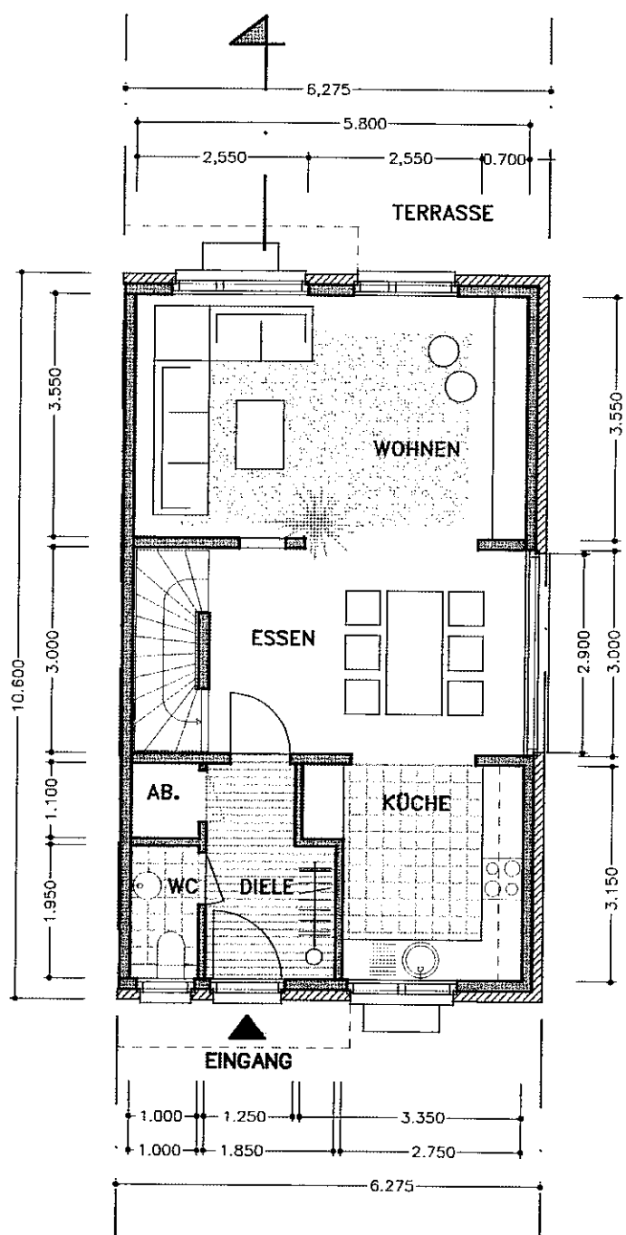
ERDGESCHOSS
