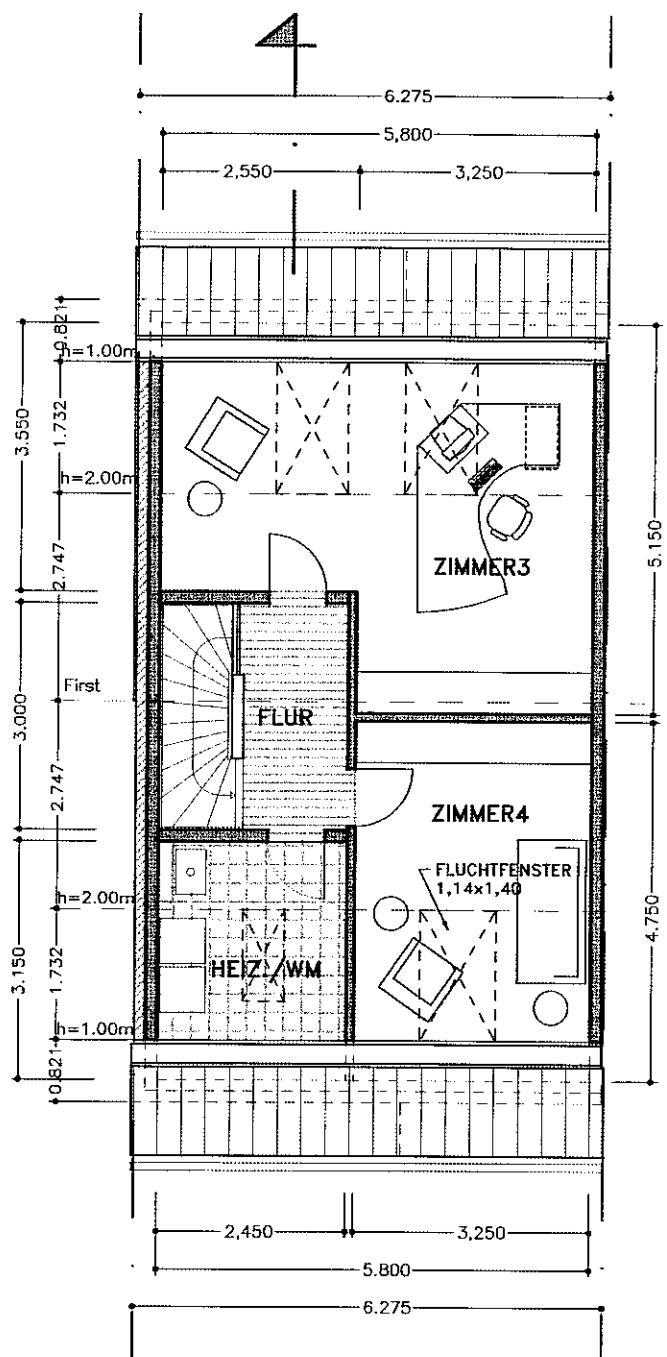
DACHGESCHOSS Sonderwunsch
