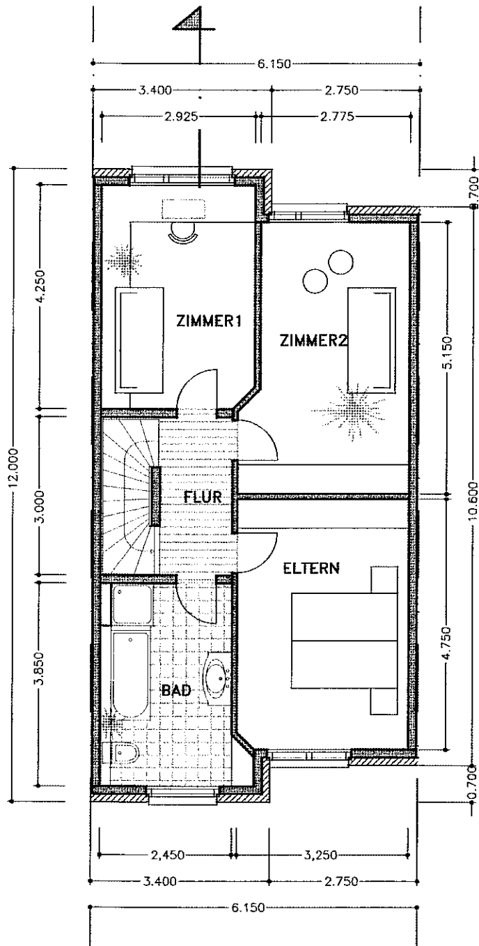
OBERGESCHOSS
