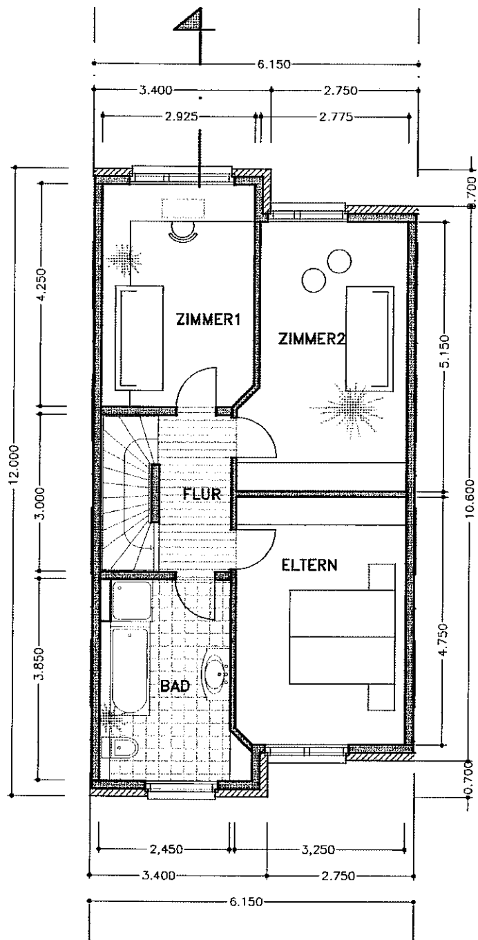
OBERGESCHOSS
