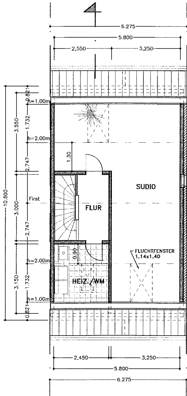
DACHGESCHOSS
