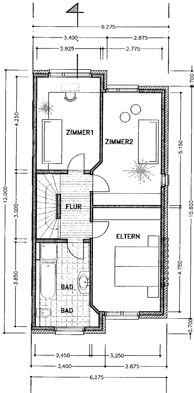
OBERGESCHOSS
