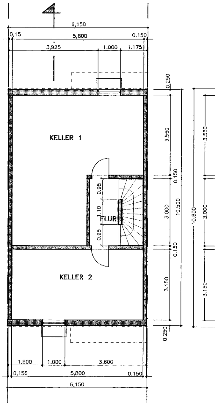
KELLERGESCHOSS
