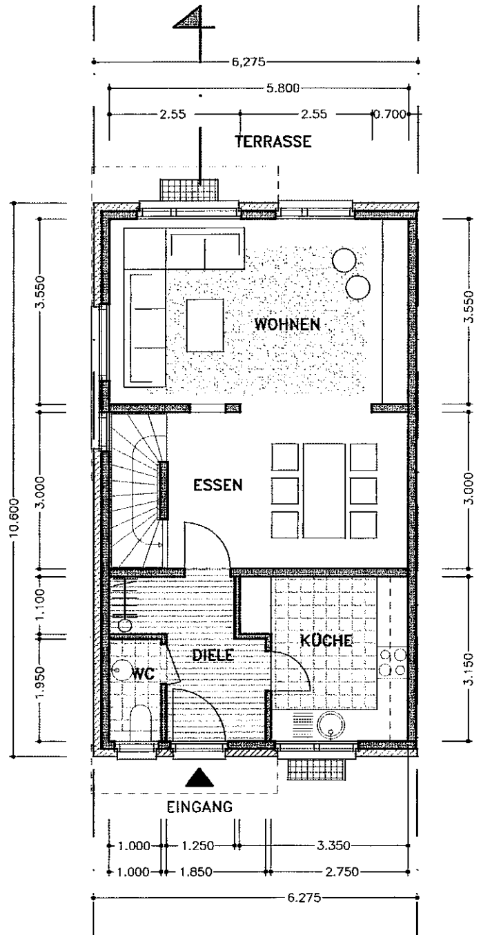
ERDGESCHOSS alternativ
