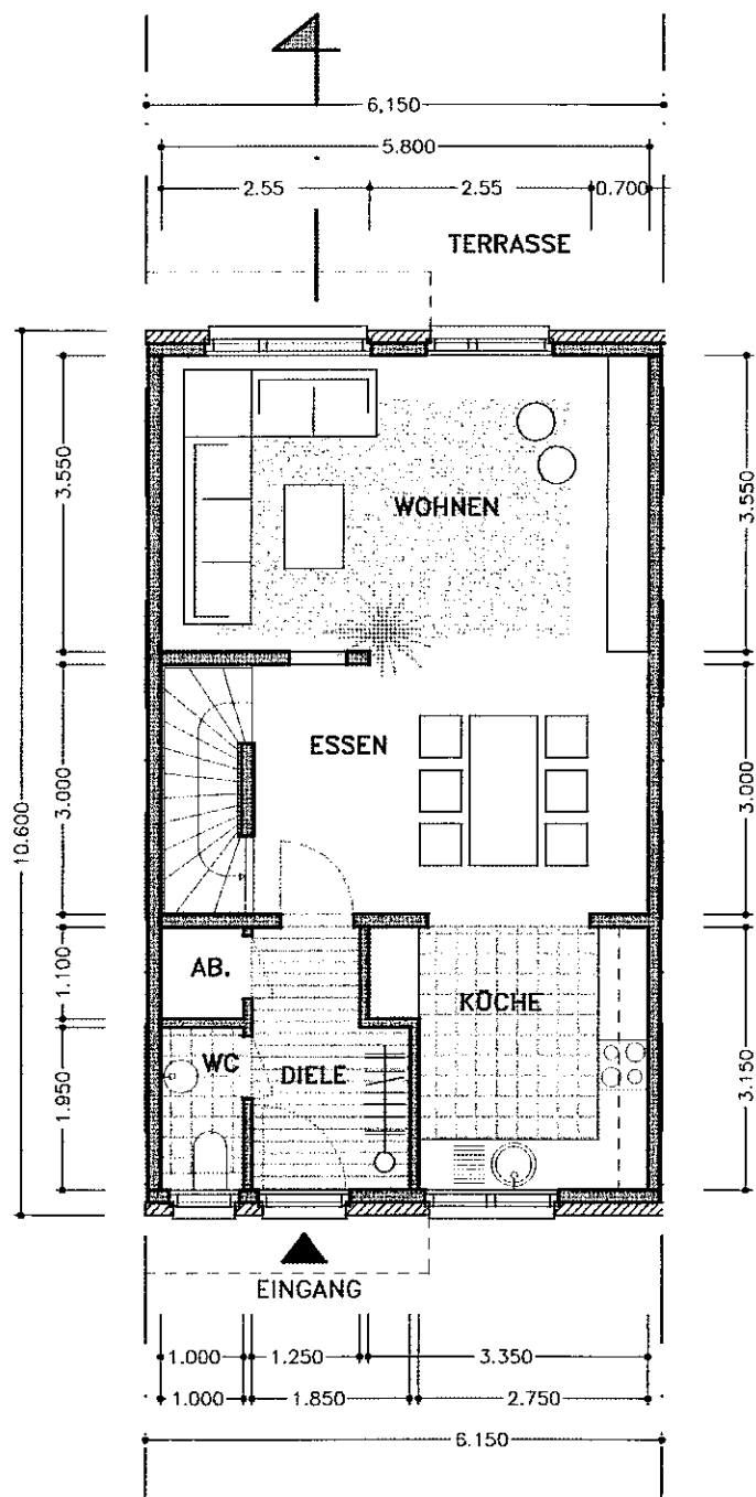
ERDGESCHOSS
