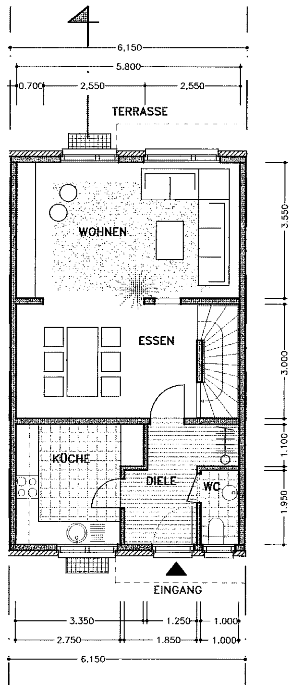
ERDGESCHOSS alternativ
