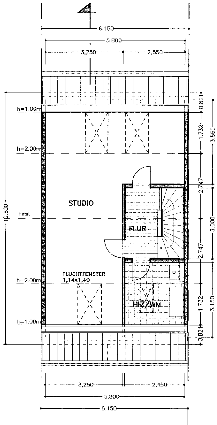
DACHGESCHOSS
