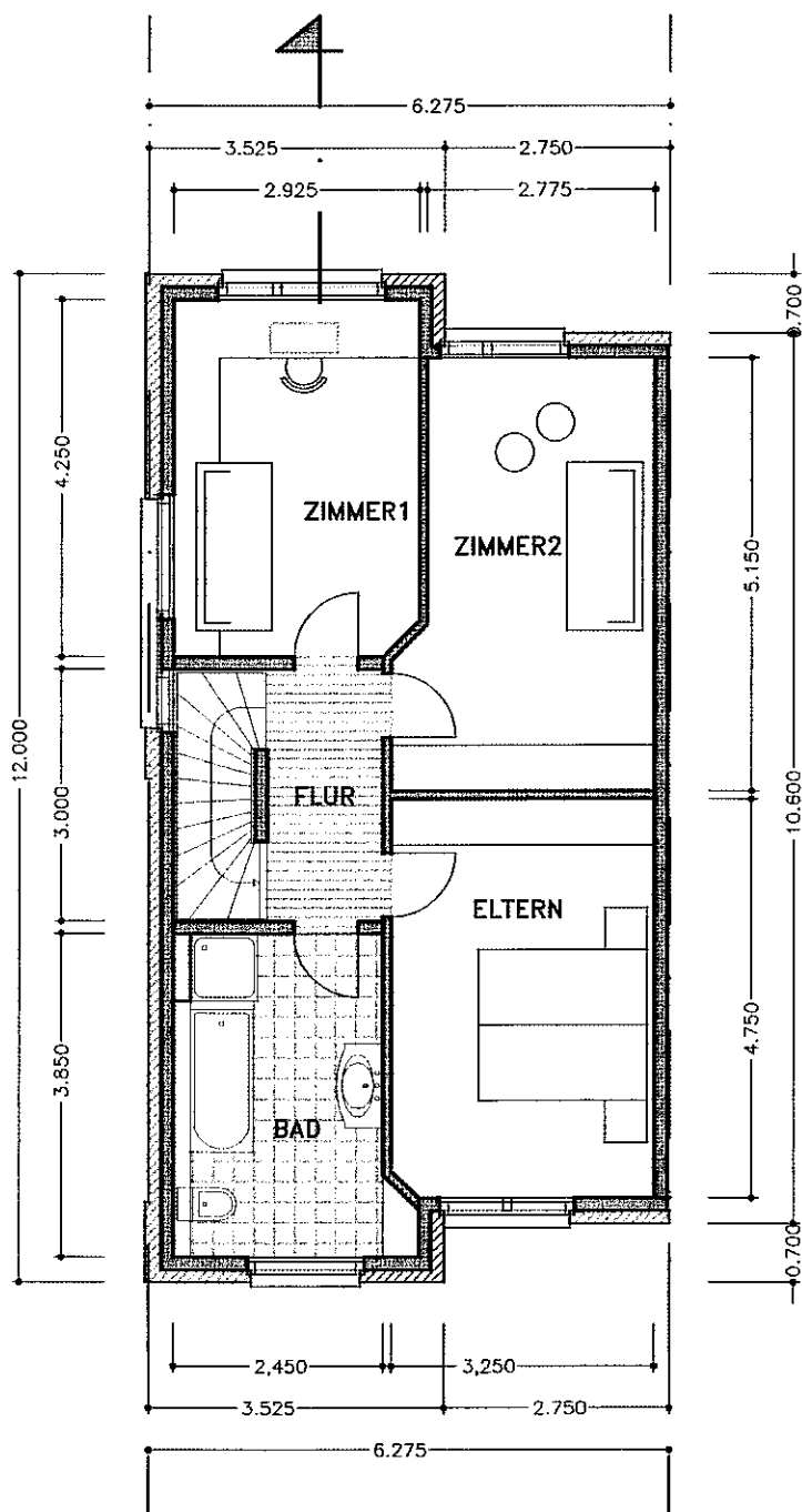
OBERGESCHOSS
