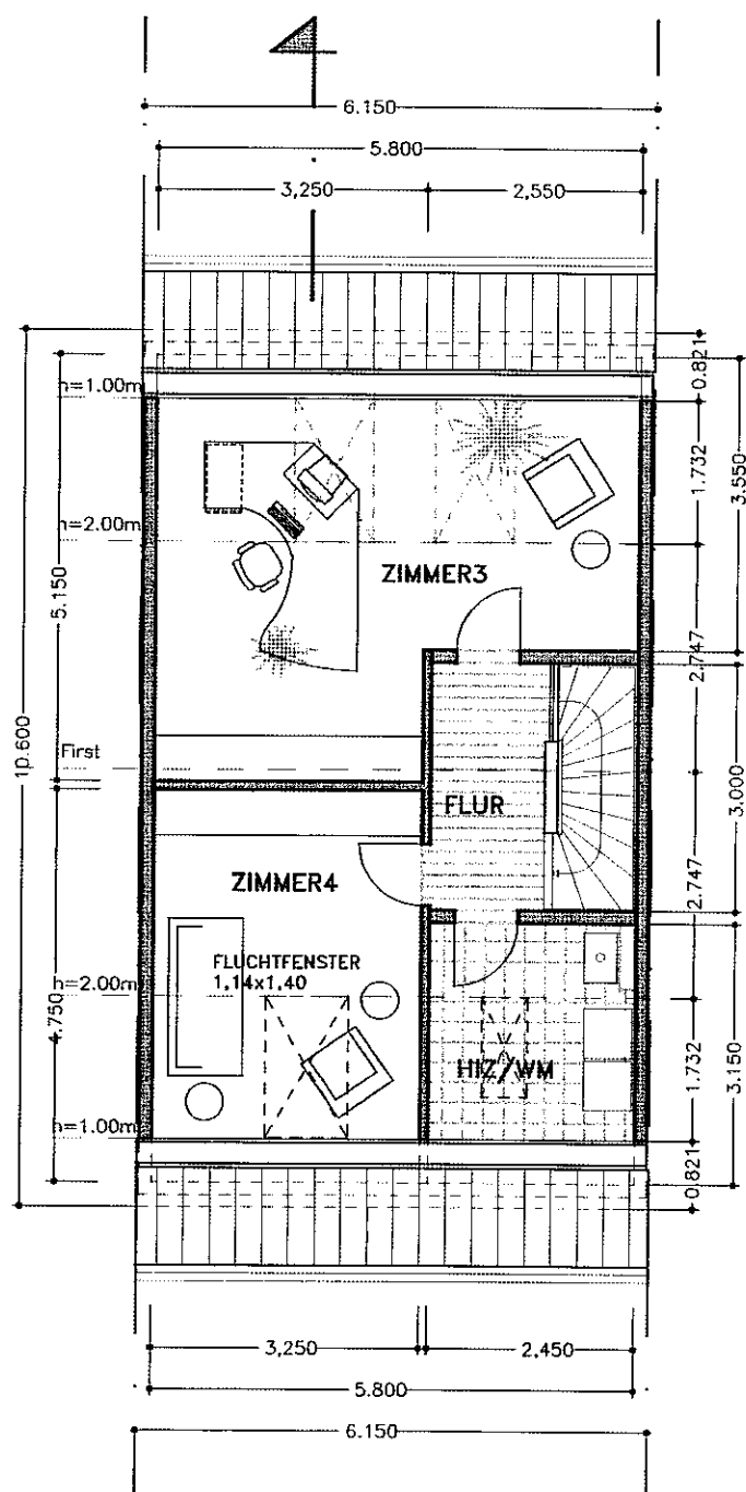
DACHGESCHOSS Sonderwunsch
