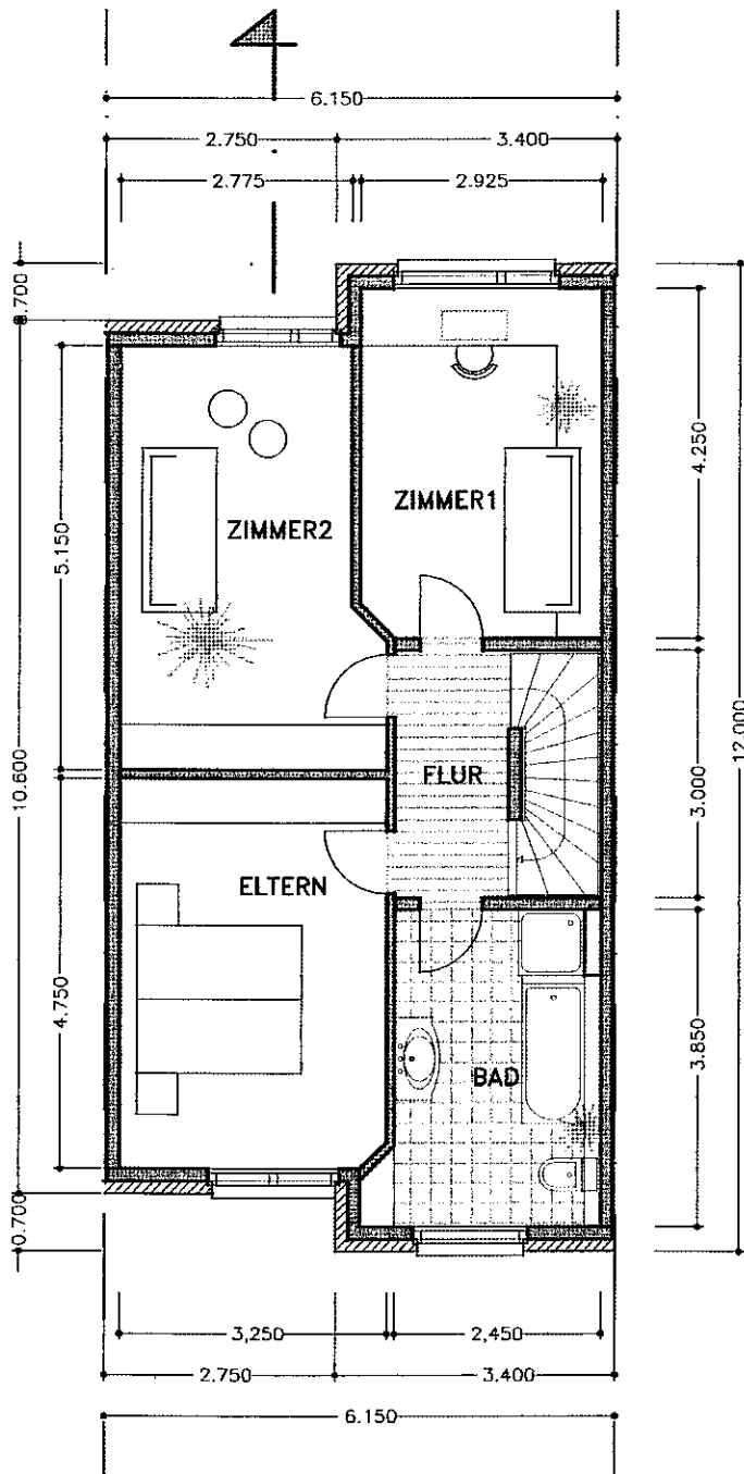
OBERGESCHOSS
