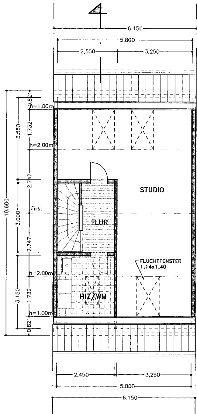
DACHGESCHOSS
