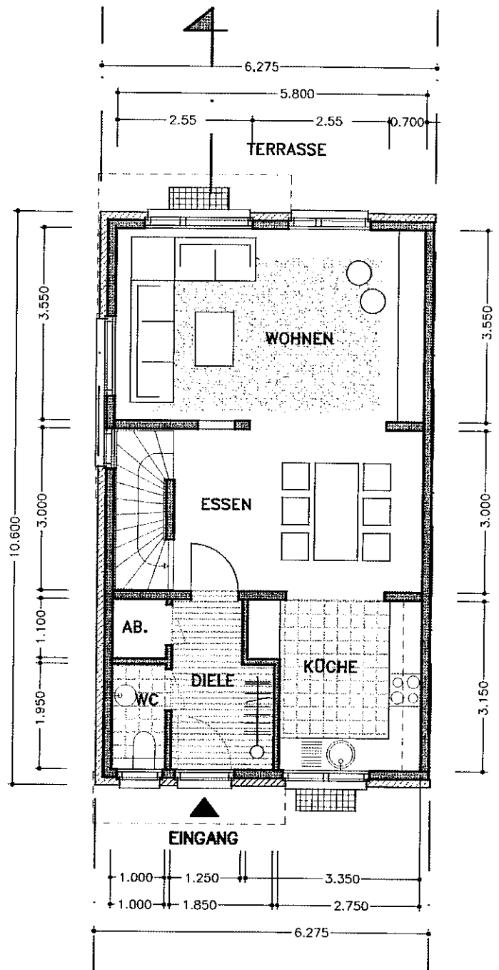
ERDGESCHOSS
