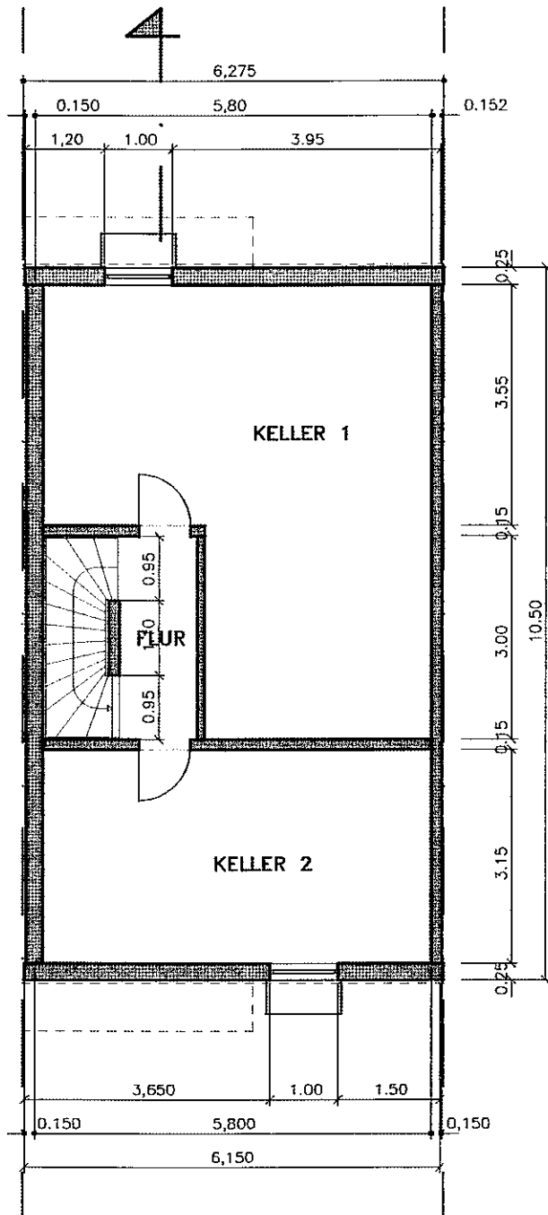
KELLERGECHOSS
