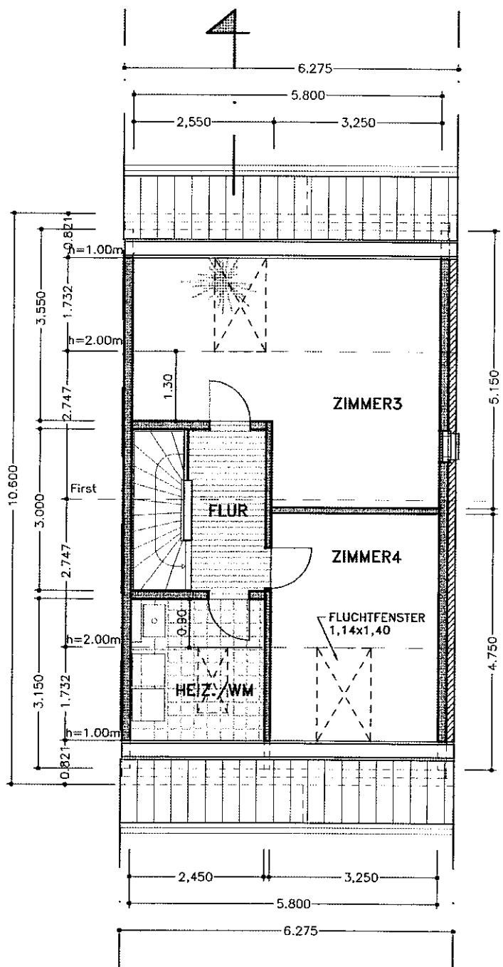
DACHGESCHOSS Sonderwunsch
