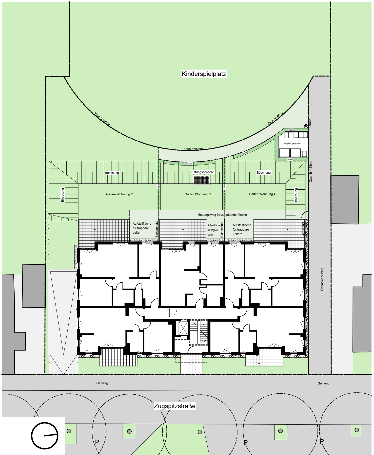
Erdgeschoss/Aussenanlage
